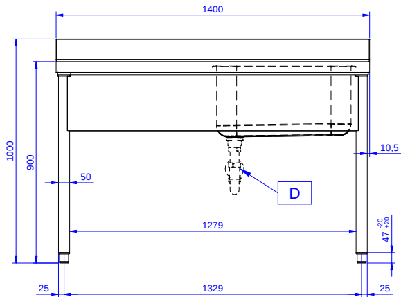
Alzado
