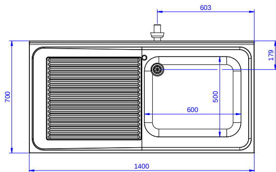
Planta
